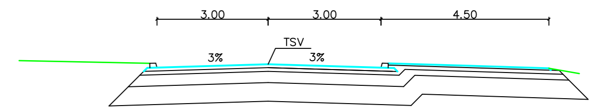
POIKKILEIKKAUS 1:100 PL 140-155
