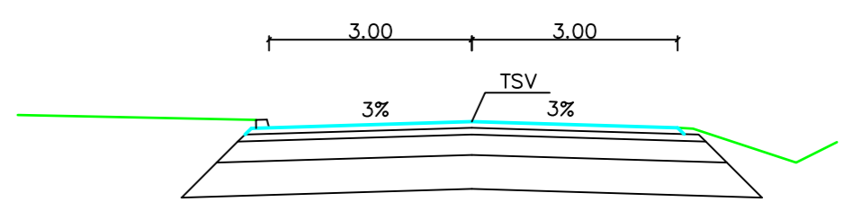
POIKKILEIKKAUS 1:100 PL 155-280
