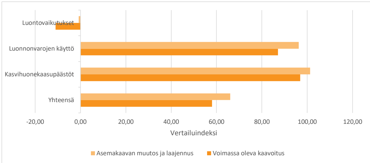
Kuva 9. Kokonaisekotehokkuus. Muokattu lähteestä KEKO, kaavoituksen ecolaskuri.
