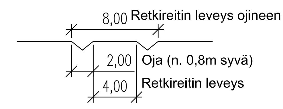
Poikkileikkaus A-A (1:200)
