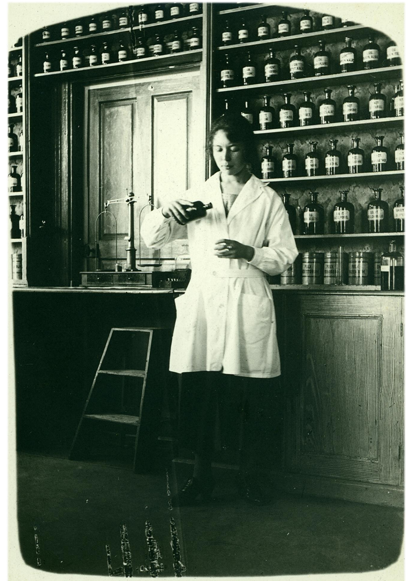
Stamapoteket på ca. 1920–30-talet. K.H. Renlunds museum.
